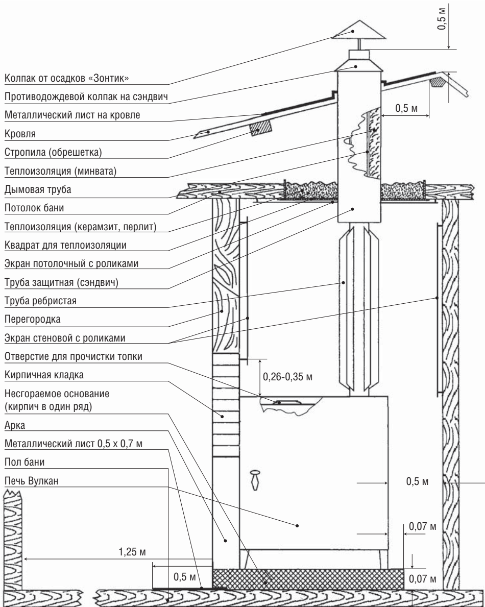
Схема монтажа и установки печи «Вулкан»
